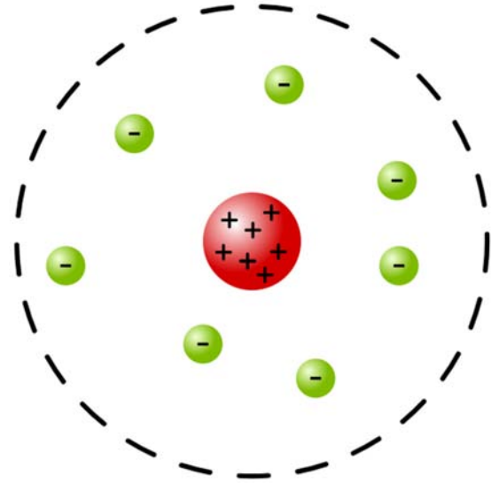
रदरफोर्डको पारमाणविक नमुना
